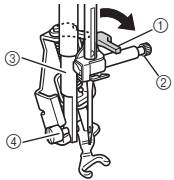
① Pino ② Parafuso de fixação da agulha ③ Barra do calçador ④ Parafuso do suporte do calçador
